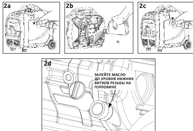
Рисунок 2 - Уровень масла
